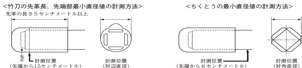
図 竹刀の先革長、先革先端部最小径値、ちくとう直径値の計測方法
